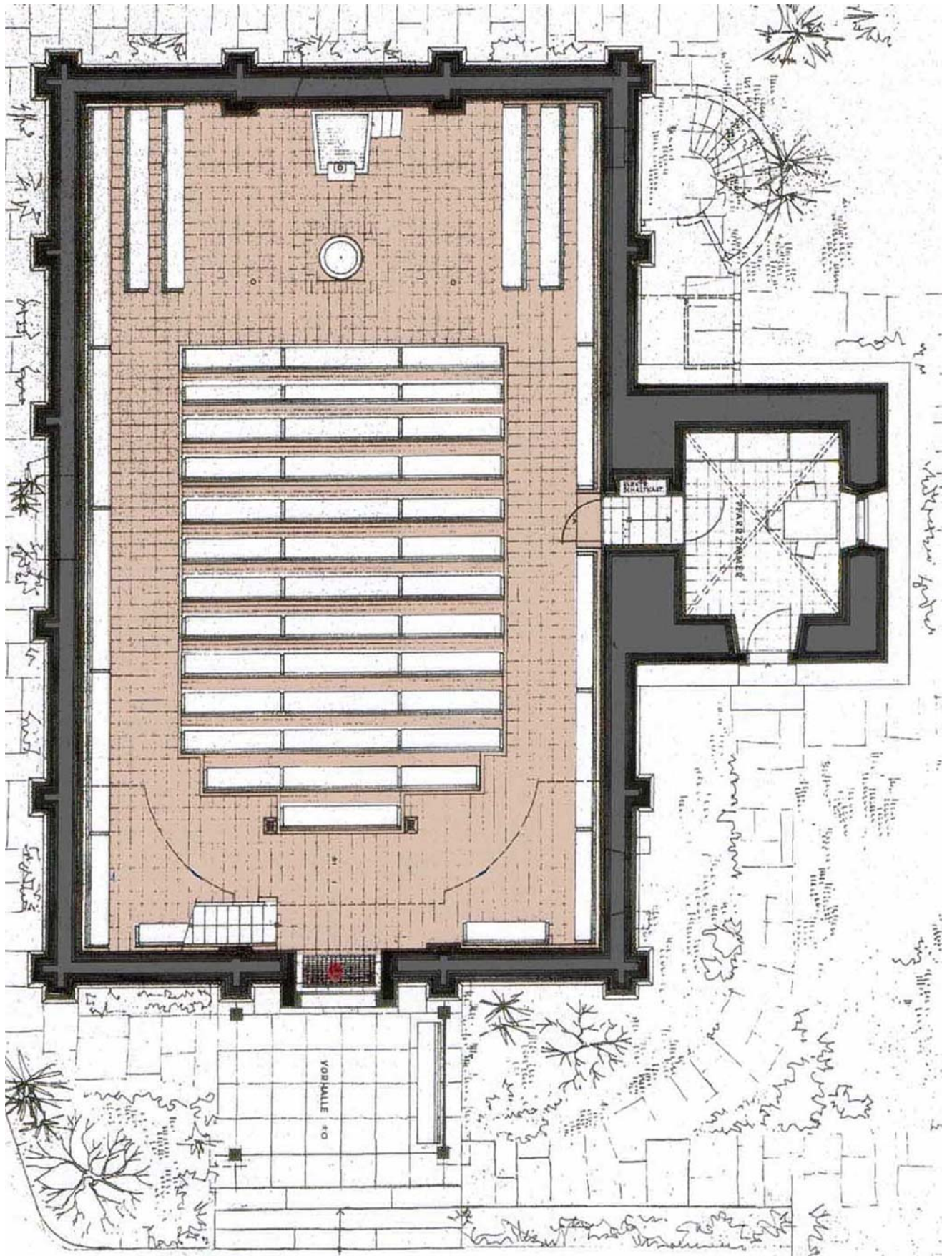
Grundriss Kirche Wangen
